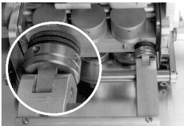
Variabel aandruk-spansysteem K9-ASS "nieuw &amp; uniek"
