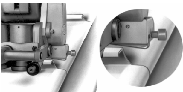
De gepatenteerde duo-veiligheidsschakelaar K9-DF, stopt de K9 automatisch bij het einde van de felsnaad of voor een muur.
