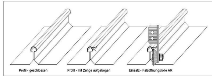
Funktion der Falzöffnungsrolle K9-1-ERB-AR
