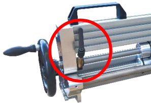
Rücklaufblockierung (standard)
