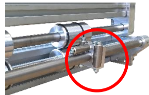
Einlaufanschlüge mit optionaler Führungsrolle und Niederhalter für die Zufuhr von Coils von oben 91263
